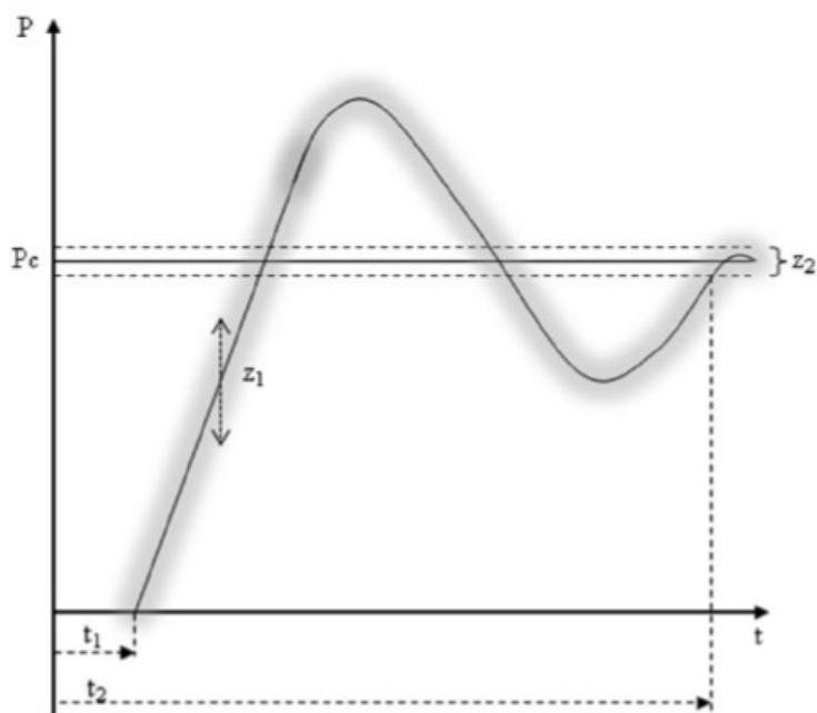
Figura nr. 4. Modul de variație a puterii active
